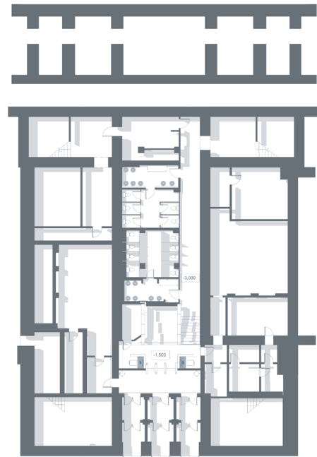
Совмещенный план на отметке -1.500 и -3.000
