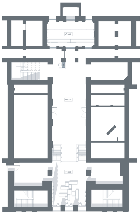
Совмещенный план на отметке 0.000 и +1.800
